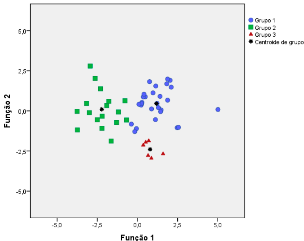
Figura 4: Centroides das funções discriminantes
