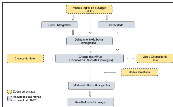
Figura 2 - Fluxograma das etapas de modelagem (SWAT). Fonte: Adaptado de Srinivas e Gopal (2017).
