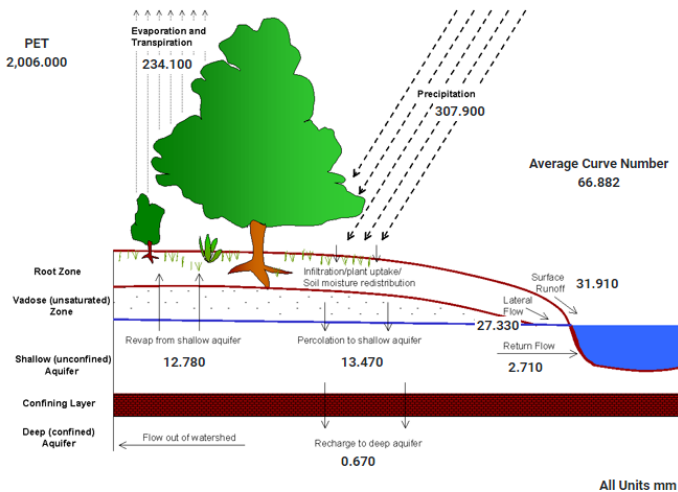
Figura 17- Balanço hídrico médio anual da bacia hidrográfica do Pontal.
