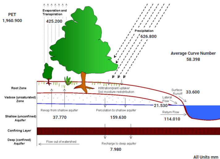
Figura 6- Balanço hídrico médio anual da bacia hidrográfica do Moxotó.
