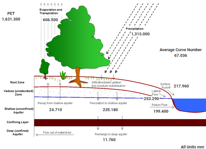
Figura 24- Balanço hídrico médio anual da bacia hidrográfica do Goiana.
