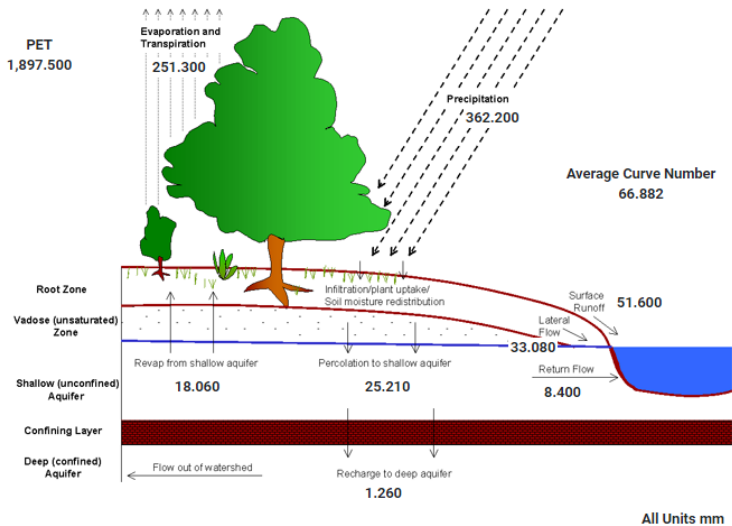
Figura 4- Balanço hídrico médio anual da bacia hidrográfica do Pontal.
