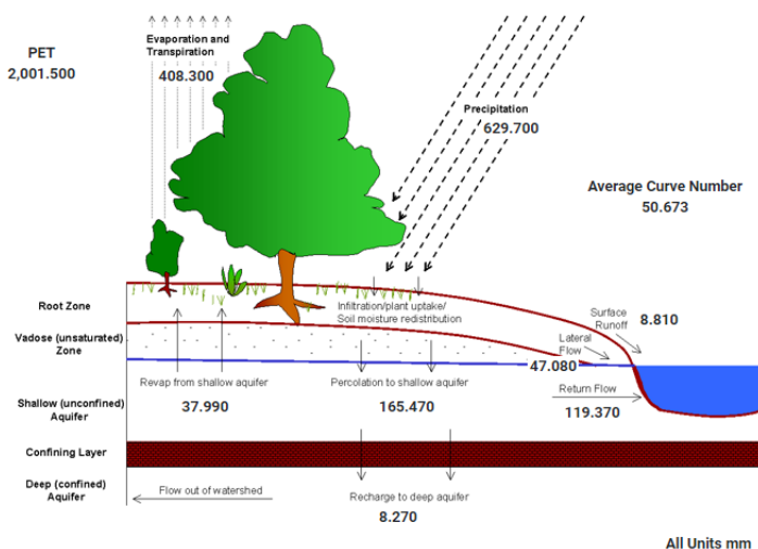
Figura 12- Balanço hídrico médio anual da bacia hidrográfica do Ipanema.
