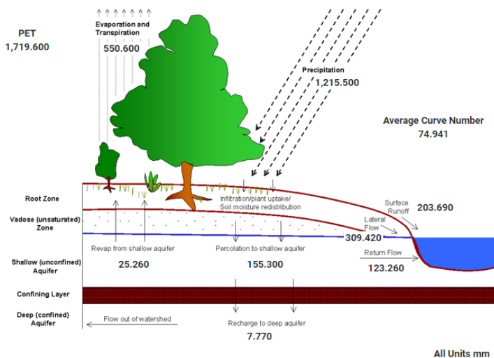
Figura 25- Balanço hídrico médio anual da bacia hidrográfica do Goiana.
