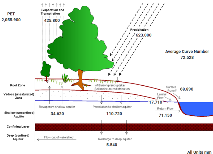
Figura 19- Balanço hídrico médio anual da bacia hidrográfica do Pajeú.
