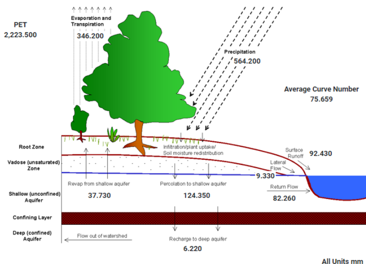
Figura 5- Balanço hídrico médio anual da bacia hidrográfica do Brígida.
