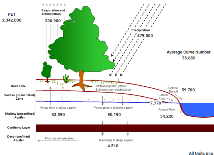
Figura 18- Balanço hídrico médio anual da bacia hidrográfica do Brígida.
