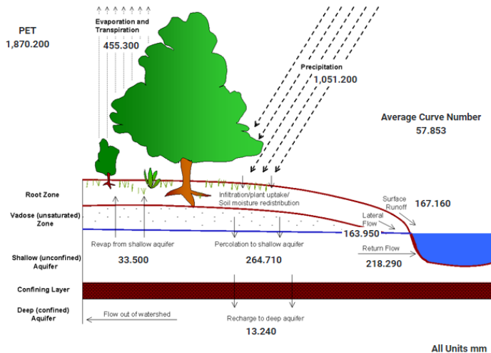
Figura 16- Balanço hídrico médio anual da bacia hidrográfica de Ipojuca.
