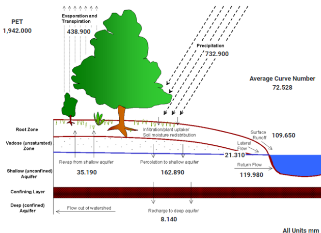
Figura 11- Balanço hídrico médio anual da bacia hidrográfica do Pajeú.
