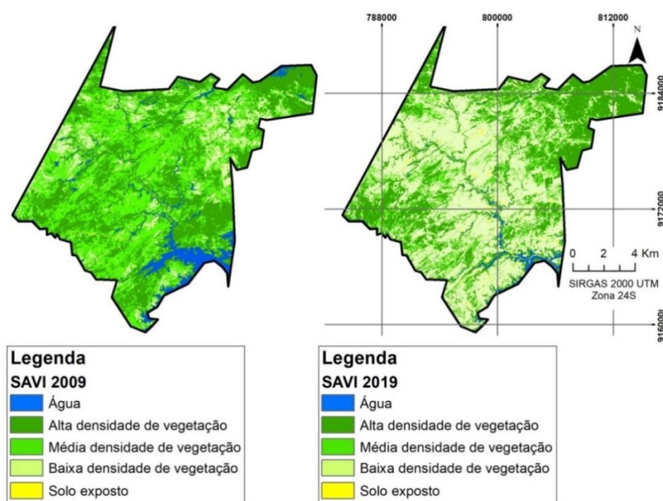
Figura 9 - Recortes temporais utilizando SAVI nos períodos (2009 e 2019) do Município de Cabaceiras-PB Fonte: Autor (2021).
