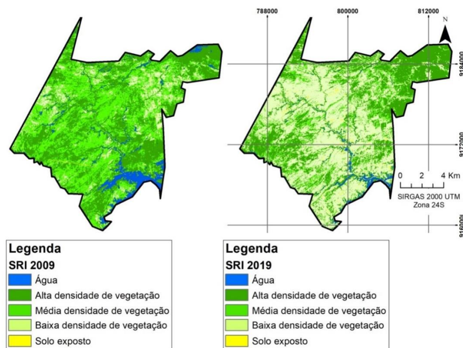
Figura 10 - Recortes temporais utilizando SRI nos períodos (2009 e 2019) do Município de Cabaceiras-PB Fonte: Autor (2021).
