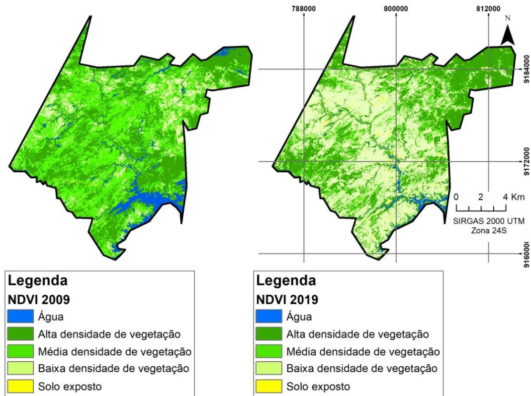
Figura 8 - Recortes temporais utilizando NDVI nos períodos (2009 e 2019) do Município de Cabaceiras-PB Fonte: Autor (2021).
