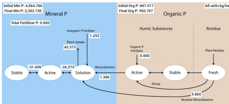
Figura 20 - Balanço de fósforo médio anual da bacia hidrográfica do Mundaú.
