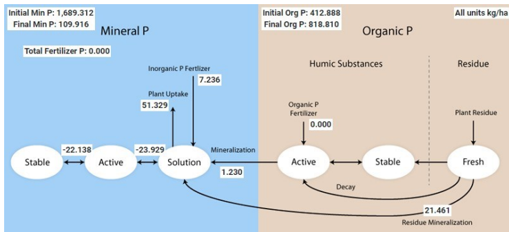
Figura 17 - Balanço de fósforo médio anual da bacia hidrográfica do Moxotó.
