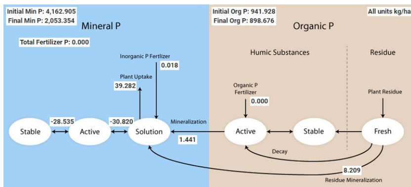
Figura 24 - Balanço de fósforo médio anual da bacia hidrográfica do Sirinhaém.
