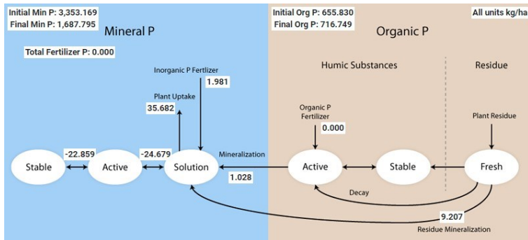
Figura 16 - Balanço de fósforo médio anual da bacia hidrográfica do Una.
