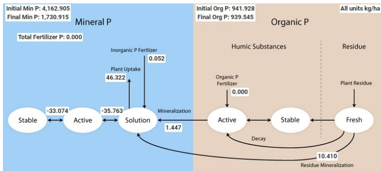
Figura 11 - Balanço de fósforo médio anual da bacia hidrográfica do Sirinhaém.
