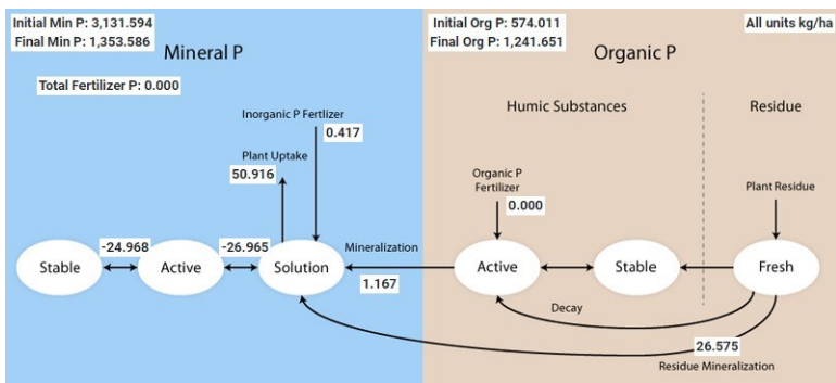
Figura 21 - Balanço de fósforo médio anual da bacia hidrográfica do Garças.
