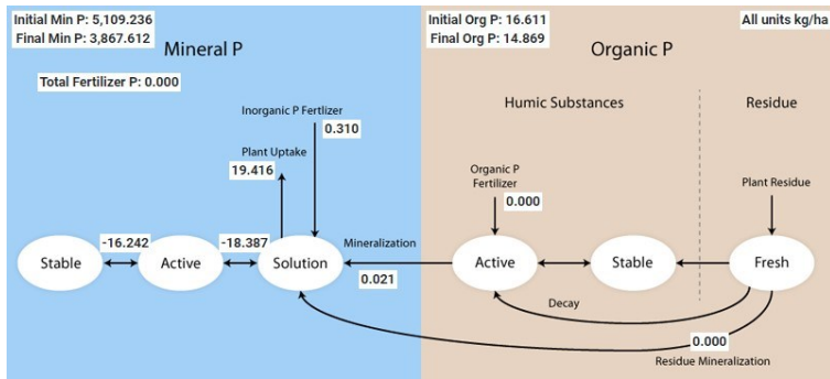
Figura 13 - Balanço de fósforo médio anual da bacia hidrográfica do Pontal.
