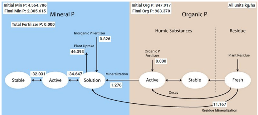
Figura 7 - Balanço de fósforo médio anual da bacia hidrográfica do Goiana.
