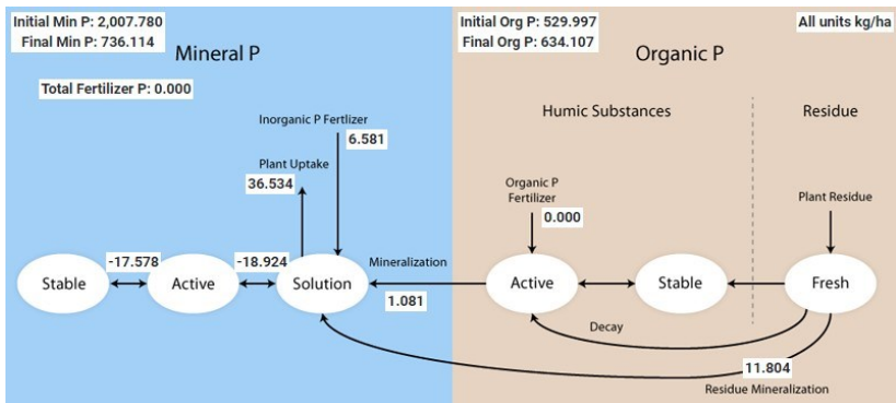
Figura 25 - Balanço de fósforo médio anual da bacia hidrográfica do Ipojuca.
