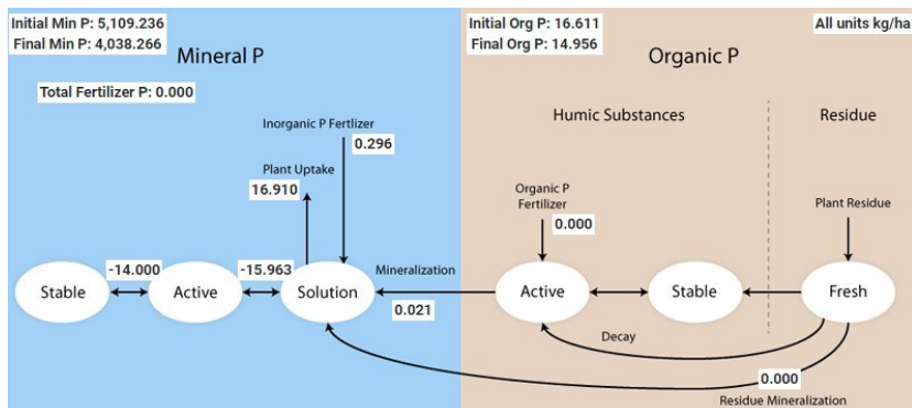
Figura 26 - Balanço de fósforo médio anual da bacia hidrográfica do Pontal.
