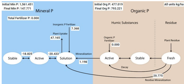
Figura 14 - Balanço de fósforo médio anual da bacia hidrográfica do Pajeú.
