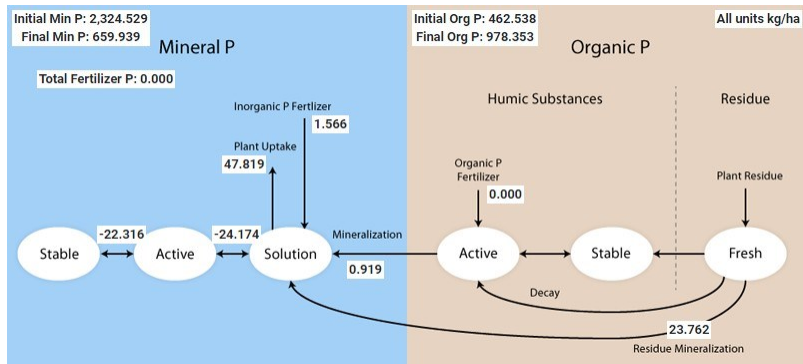
Figura 10 - Balanço de fósforo médio anual da bacia hidrográfica do Brígida.
