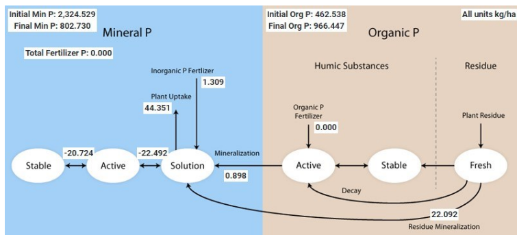
Figura 22 - Balanço de fósforo médio anual da bacia hidrográfica do Brígida.
