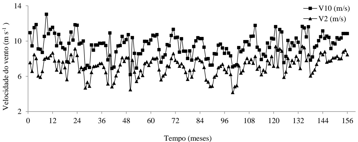
Figura 3. Variação da velocidade máxima instantânea mensal do vento a 2 m e a 10 m de altura no período de janeiro de 2000 à dezembro de 2012, em Mossoró/RN.
