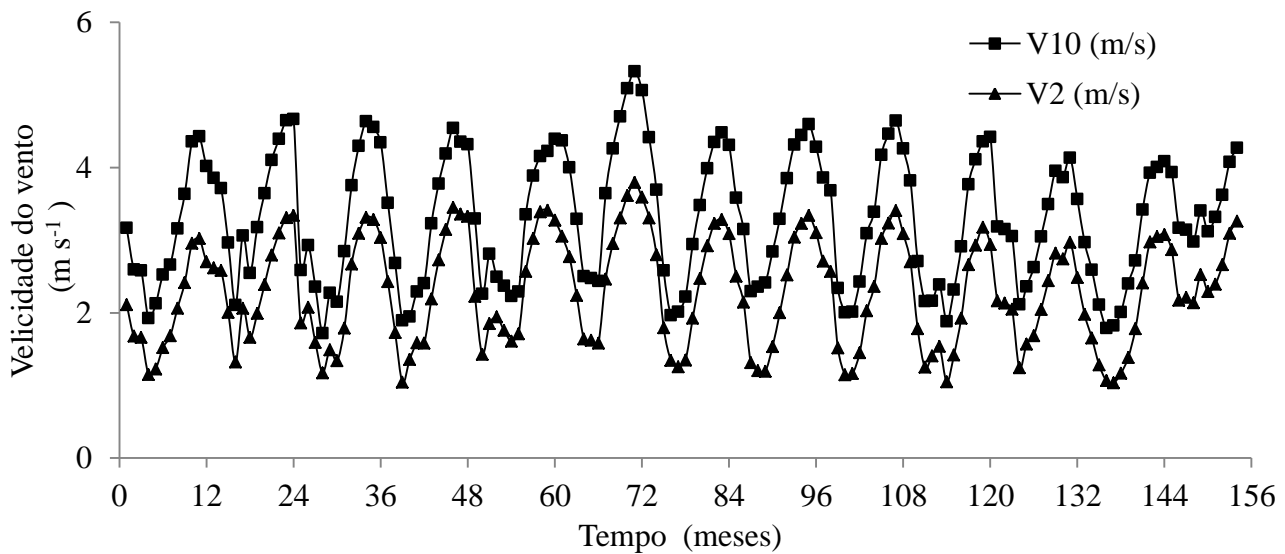
Figura 1. Variação da velocidade média mensal do vento a 2 m e a 10 m de altura no período de janeiro de 2000 a dezembro de 2012 em Mossoró/RN.
