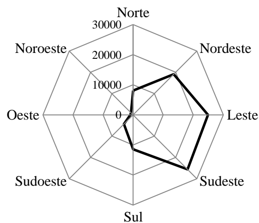
Figura 4. Frequência média anual da direção do vento, no período de 2000 à 2012, em Mossoró/RN.
