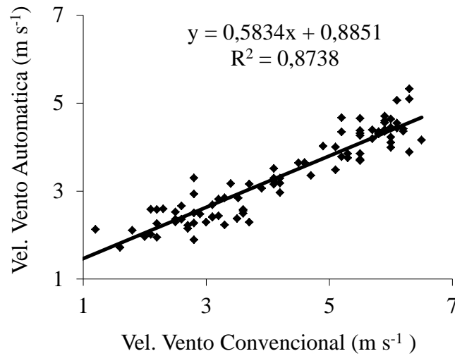
Figura 2. Correlação da velocidade do vento ( m s^{-1} ) da estação automática com a velocidade do vento ( m s^{-1} ) da estação convencional, para Mossoró/RN.
