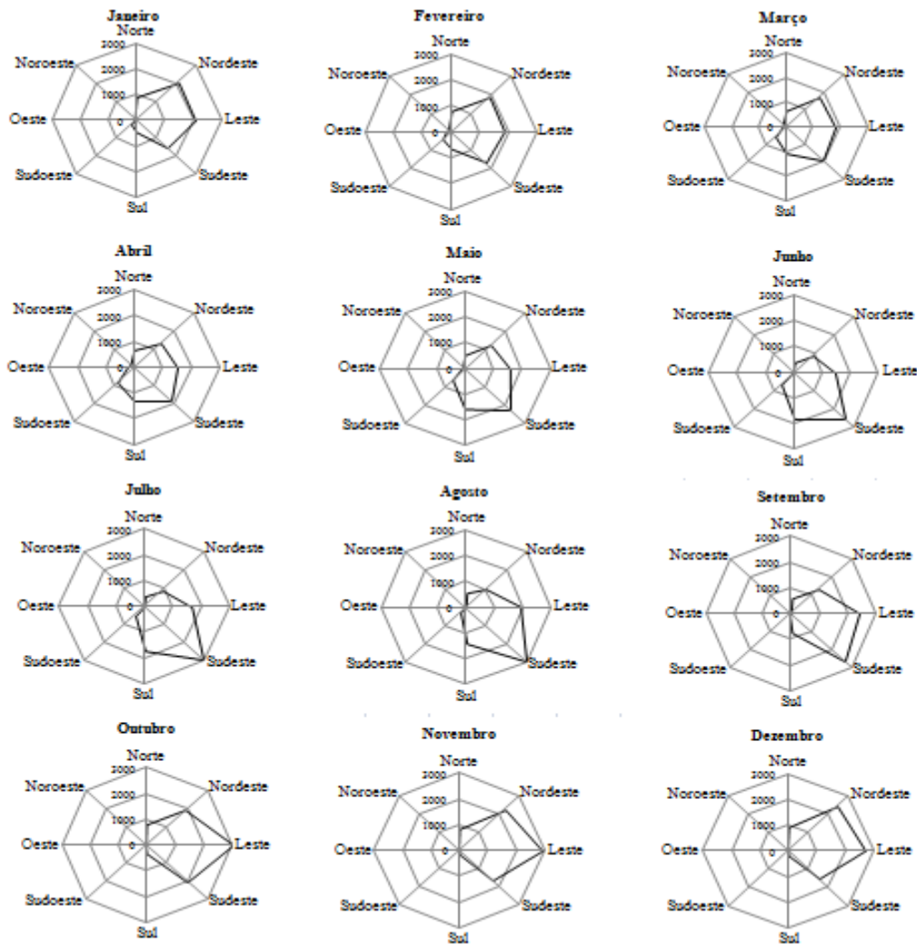
Figura 5. Frequência média da direção do vento, nos doze meses do ano, no período de janeiro de 2000 à dezembro de 2012, em Mossoró/RN.
