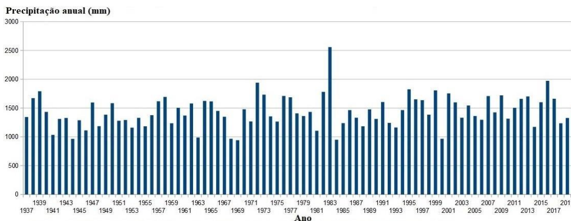
Figura 6 – pluviograma de precipitação anual da área de Araraquara para o período entre 1937 e 2020, feito com base nos dados do pluviômetro do DAAE (Departamento de Águas de Araraquara).
