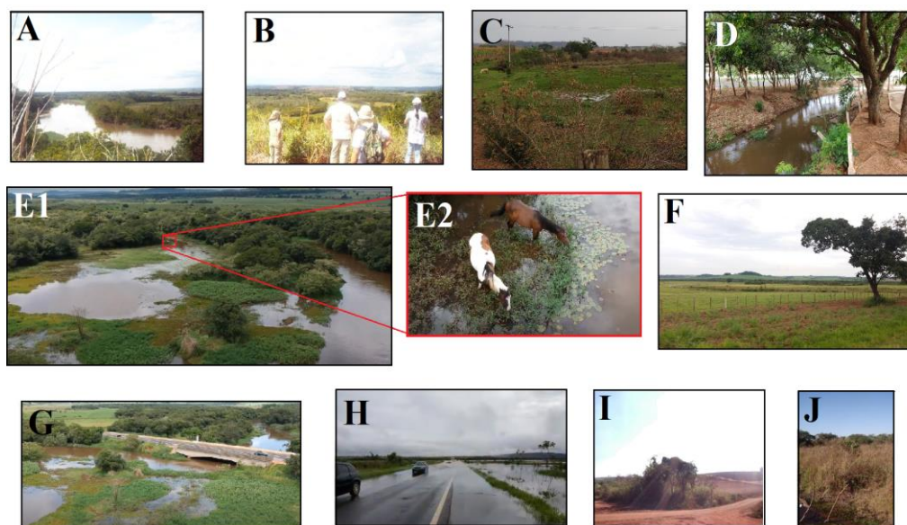
Figura 20 – composição de fotografias das Terras Baixas: A – meandro do Rio Mogi-Guaçu e sua planície aluvial no município de Rincão; B: planície aluvial do rio Mogi-Guaçu e seus meandros abandonados também no município de Rincão; C – planície aluvial do rio Boa Esperança, usada para pastagem, no município de Trabiçu; D: rio Boa Esperança no trecho em que sua planície aluvial foi sobreposta por um segmento da mancha urbana de Boa Esperança do Sul; E: Rio Jacaré-Guaçu e sua planície de inundação logo após uma das recorrentes inundações da mesma – em E2 vê-se detalhe de cavalos que ali pastavam antes da inundação e ficaram momentaneamente envolvidos pelas águas extravasadas pelo rio; F: baixos terraços do rio Jacaré-Guaçu no município de Boa Esperança do Sul, área que é atingida por extravasamento das águas do rio apenas em momentos de chuvas extraordinariamente intensas; G: ponte da rodovia Comandante Barros cruzando o Rio Jacaré-Guaçu e parte de sua planície de inundação; H: trecho da supracitada rodovia sendo recoberto pelas águas de inundações do rio Jacaré-Guaçu; I e J: afluente assoreado do Ribeirão das Cruzes, no município de Santa Lucia. Fonte: fotografias próprias, e imagens de drone de Higor Vanessa.
