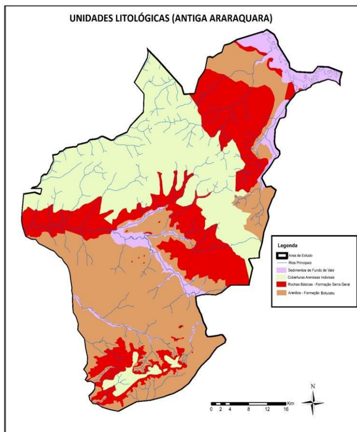
Figura 4 – mapa das unidades geológicas
