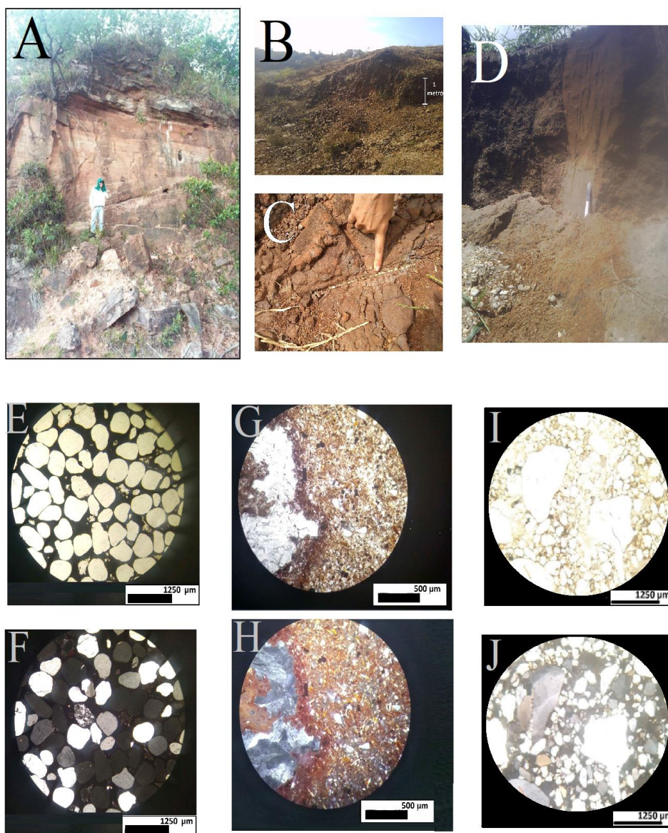
Figura 5 – afloramentos representativos das principais unidades geológicas, e capturas microfotográficas representativas de suas principais características petrográficas: A – afloramento de arenitos da Fm. Botucatu, no município de Santa Lucia; B – afloramento de basaltos da Fm. Serra Geral, no município de Dourado, C: detalhe apontado fraturas em rochas ígneas básicas, parte delas preenchidas por veios de materiais silicosos, no município de Américo Brasiliense, D: depósitos arenosos de fundo de vale adjacente ao Ribeirão Anhumas, em seu médio curso; E e F: microfotografias de arenitos da Fm. Botucatu, com nicois cruzados e descruzados, respectivamente – manchas escuras são constituídas por resina usada para impregnar a amostra, evidenciando a elevada porosidade que usualmente as caracteriza; G e H: microfotografias de rochas básicas da Fm. Serra Geral, com nicois cruzados e descruzados, respectivamente – a direita vemos o padrão predominante em tais rochas, de minerais de granulação fina dispostos adjacentes uns aos outros e sem formação de poros entre eles, a esquerda vemos padrão menos usual – presença de pontuais minerais de granulação muito maior que o usual de tais rochas; I e J: microfotografias de depósitos arenosos de fundo de Vale das Terras Baixas, nicois cruzados e descruzados, respectivamente. Adaptado de fotografias de acervo pessoal, Cheliz (2011) e de Cheliz (não publicado).
