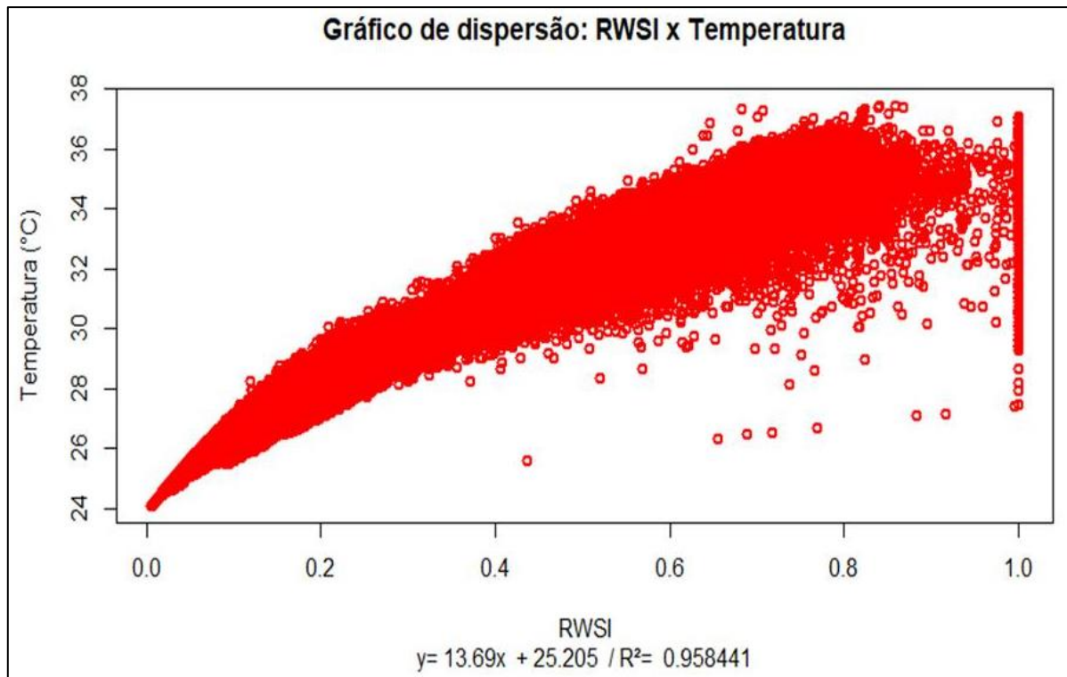
Figura 4: Gráfico da correlação entre o Índice de Estresse Hídrico Regional (RWSI - Regional Water Stress Index ) e a Temperatura da Superfície ( T_s ), na área de estudo.
