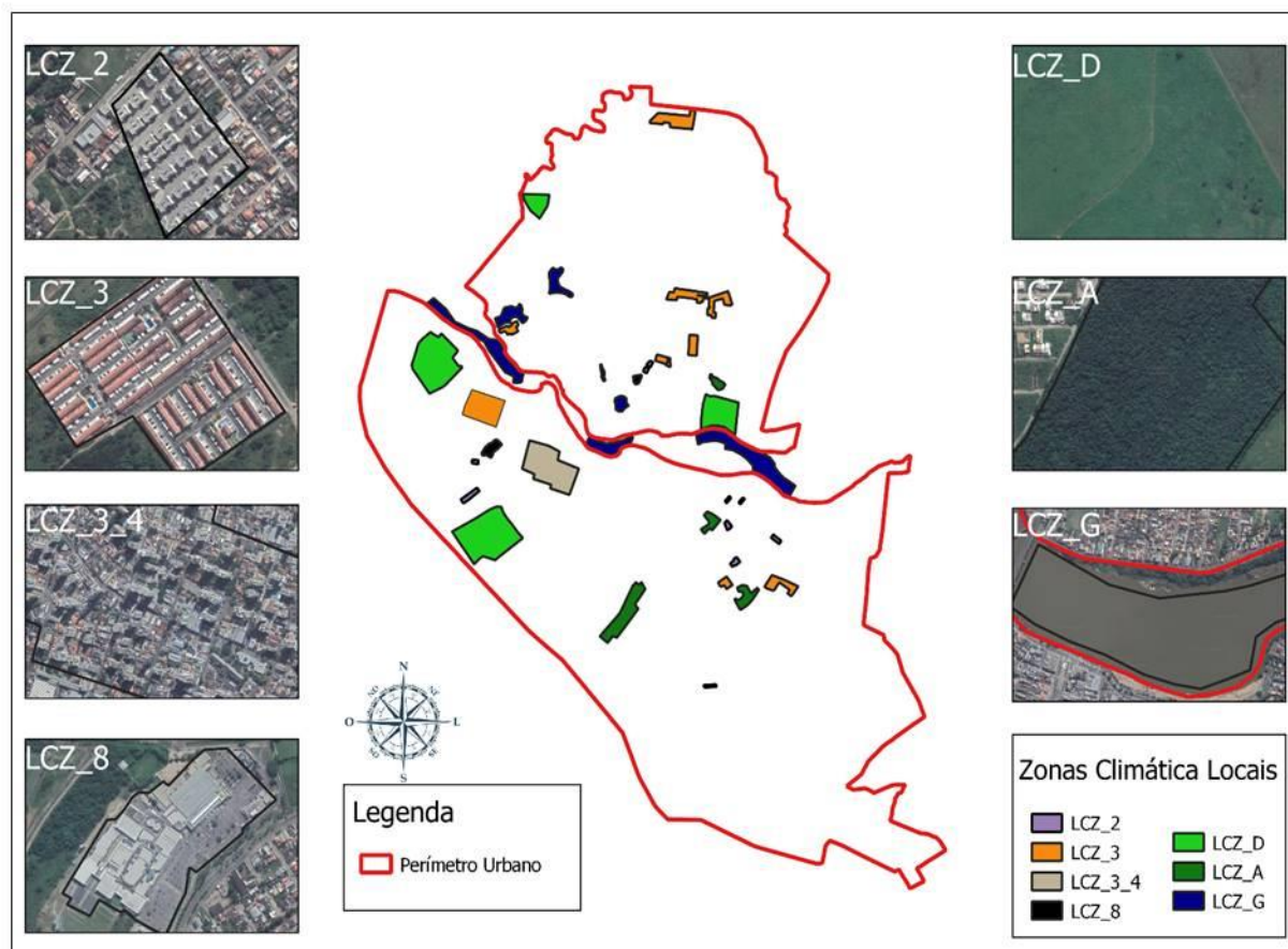
Figura 2: Localização das 8 LCZ (Zonas Climáticas Locais). Fonte: Os autores. Recortes da Imagem do Landsat 8.
