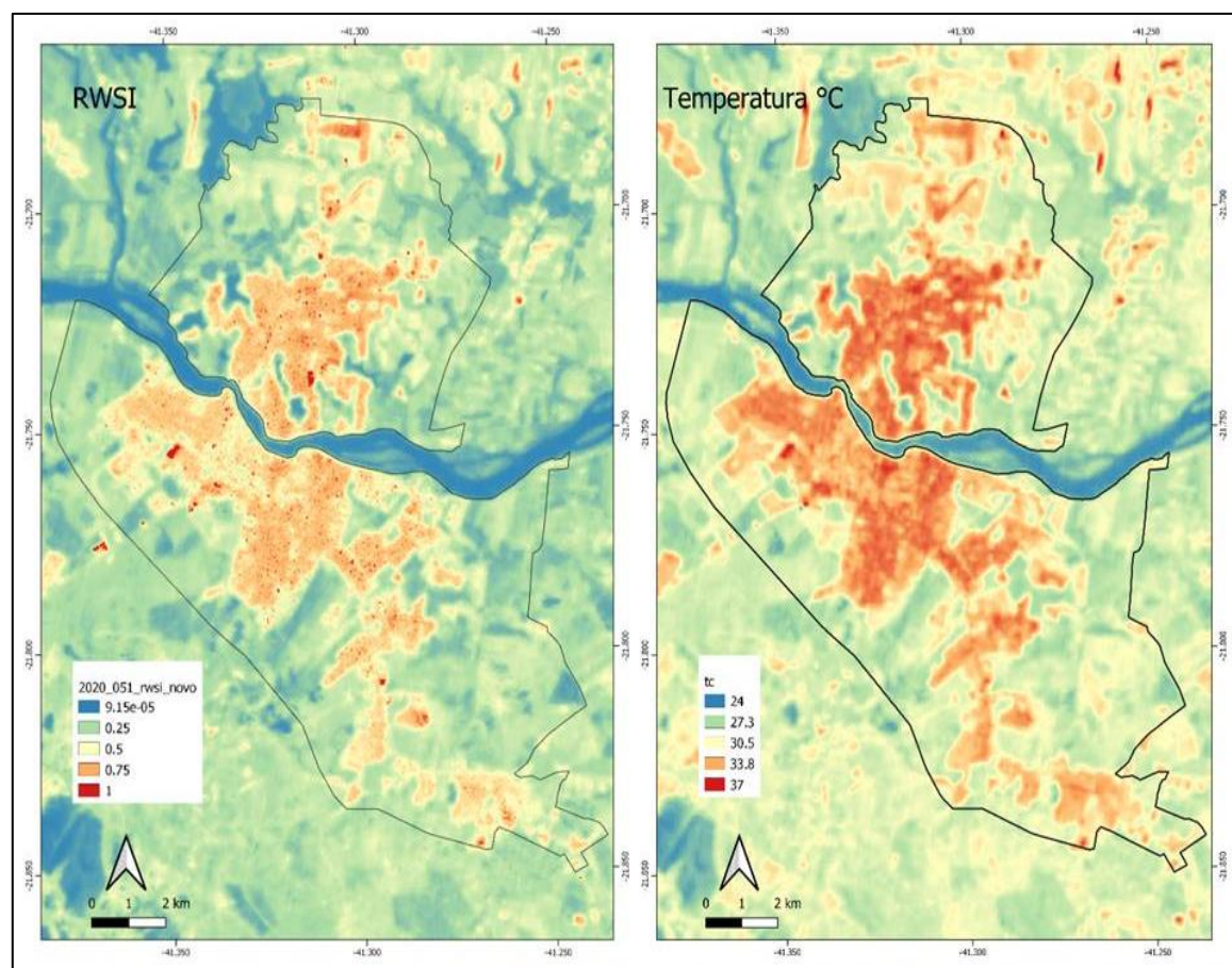
Figura 3: Apresentação das cartas dos valores do Índice de Estresse Hídrico Regional (RWSI - Regional Water Stress Index ) e da Temperatura da Superfície (Ts), na área de estudo.
