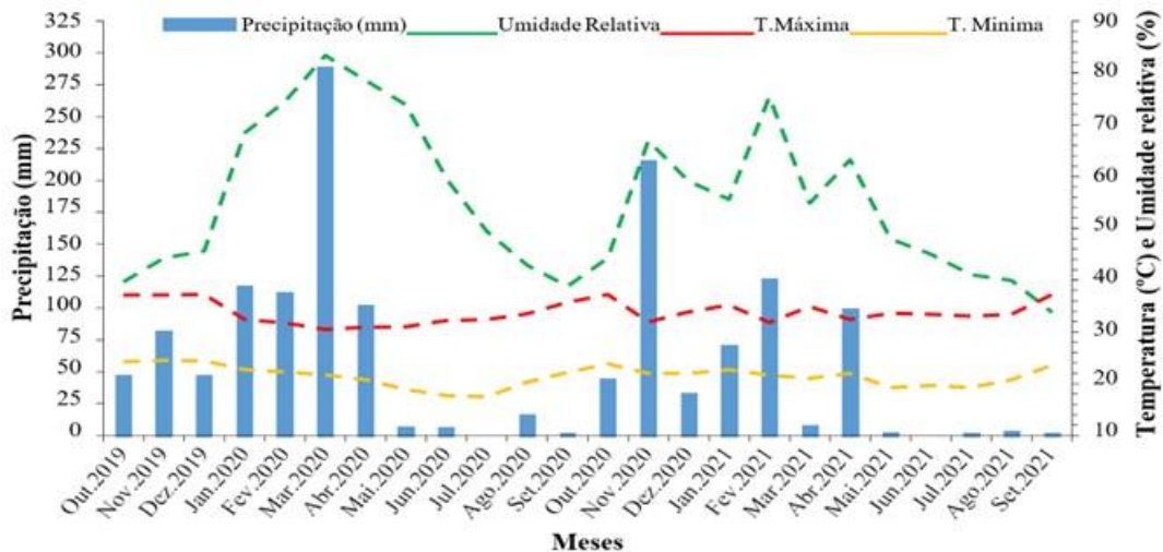
Figura 2. Precipitação mensal (mm), Umidade relativa (%), Temperatura máxima (°C) e Temperatura mínima (°C) durante o período de 01/10/2019 a 01/09/2021, registradas pela estação automática (SEIA) para o município de Paratinga-BA.
