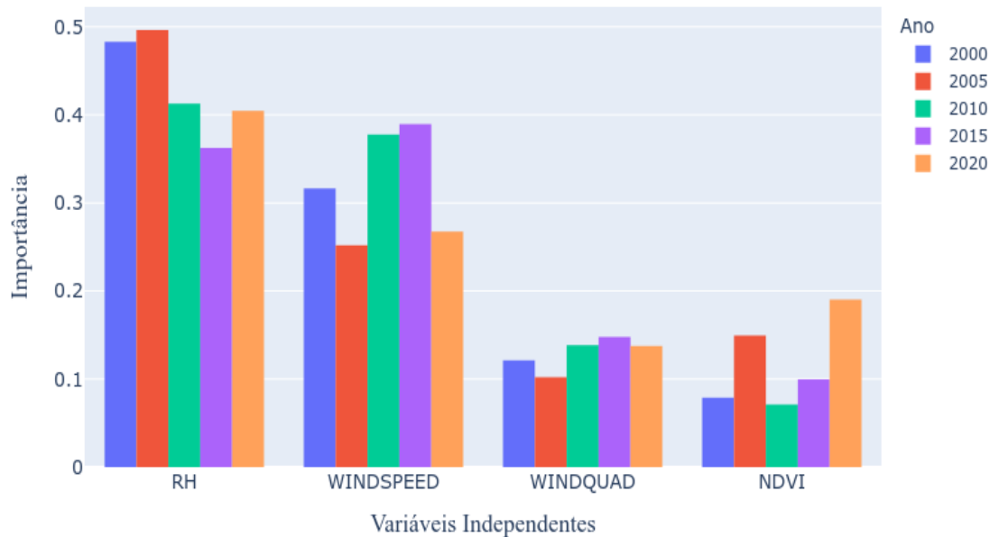
Figura 7: Classificação da importância das variáveis independentes para UTFVI em relação à superfície do solo referentes aos dados amostrais do período de 2000-2020.
