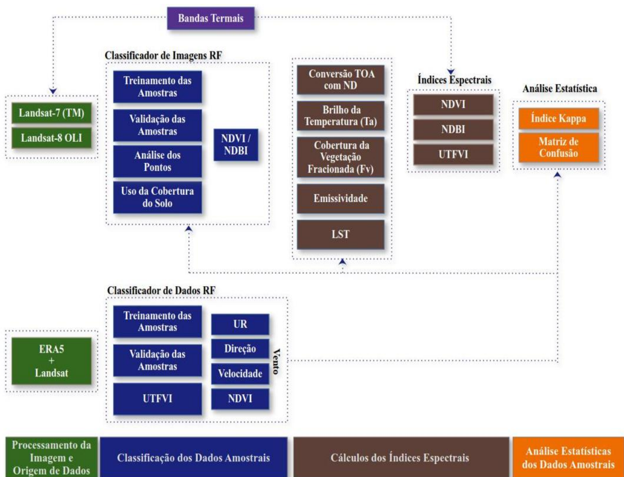
Figura 2: Fluxograma dos dados meteorológicos e pré-processamento dos dados. (Baseado em ULLAH et al., 2022).
