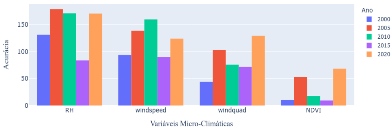
Figura 8: Médias do decréscimo da acurácia referentes ao período 2000-2020 para UTFVI a 2 metros de altura.
