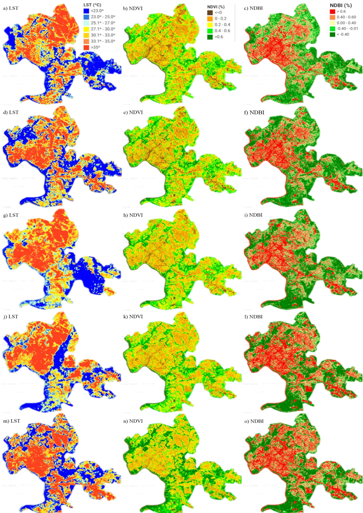
Figura 13: Os valores LST, NDVI e NDBI com variação espaço-temporal em Cuiabá-MT para o período de 2000 (a-c), 2005 (d-f), 2010 (g-i), 2015 (j-i) e 2020 (m-o).
