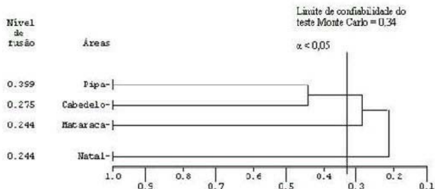
Figura 2. Dendrograma de similaridade utilizando o índice de Sørensen entre a área de Pipa, Tibau do Sul, Parque das Dunas – RN; Cabedelo – João Pessoa, Mataraca - PB, acompanhado do teste de permutação Monte Carlo = 0,34. \alpha = nível de significância.
