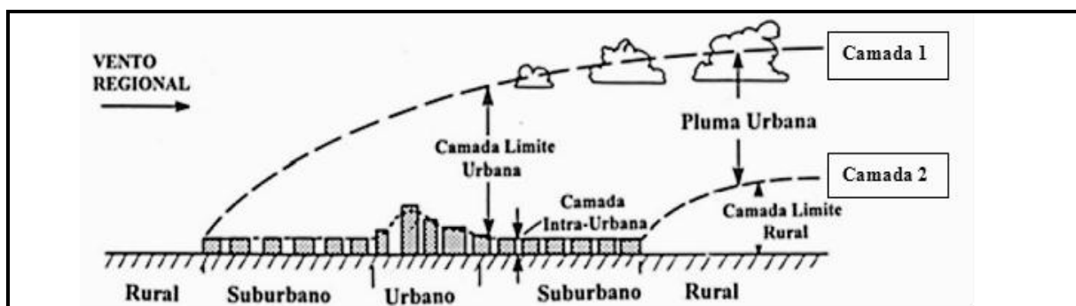
Figura 1 - Representação esquemática da atmosfera urbana. Fonte: Ilustração de OKE apresentada por Carvalho, 2001 p. 89.
