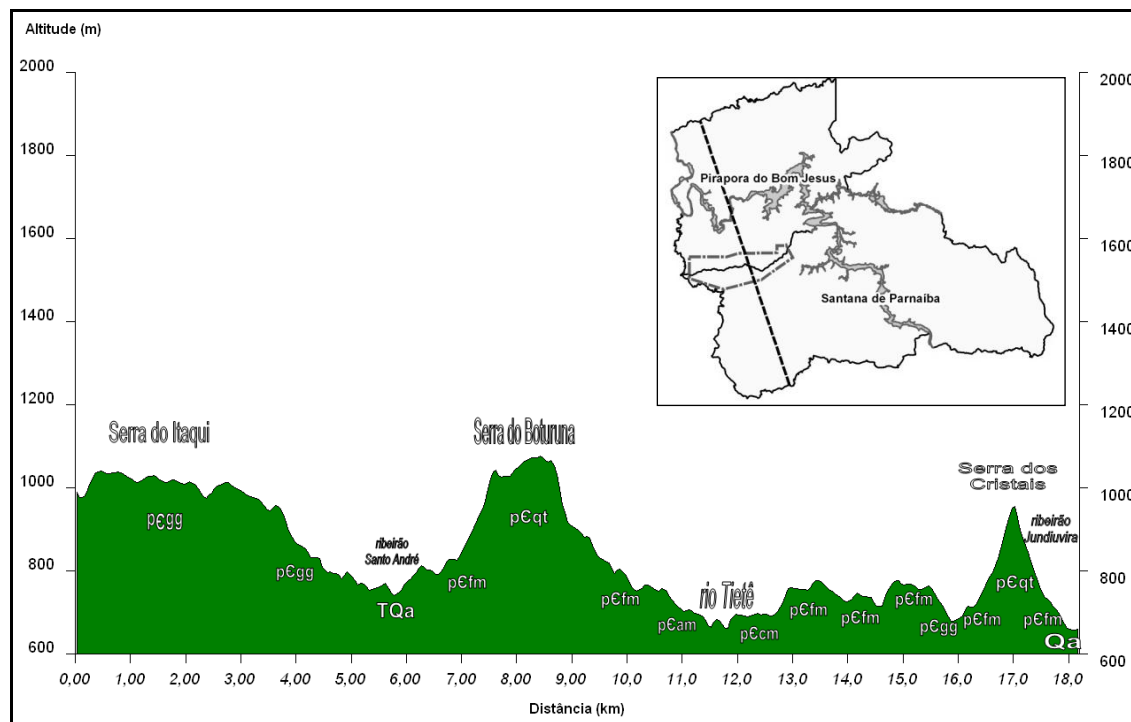
Figura 1: Perfil topográfico esquemático da região da Serra do Boturuna
