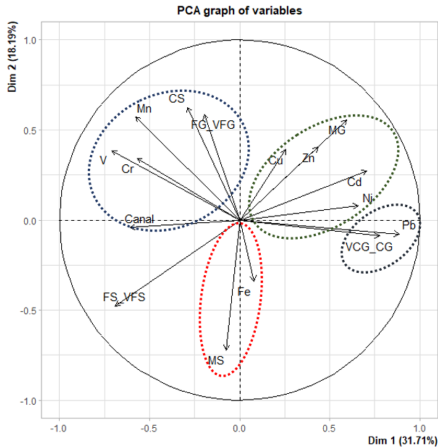
Gráfico 4 – Resultado del Análisis de Componentes Principales.
