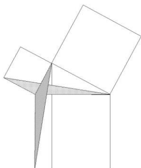
Figura 5: Diagrama de Euclides para la demostración del Teorema de Pitágoras ( Elementos , I.47)
