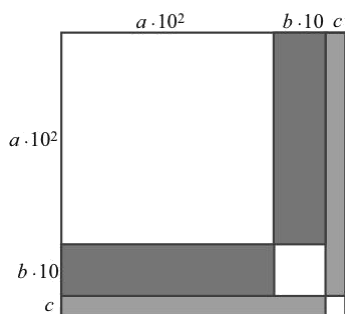
Figura 9: Interpretación geométrica de Liu Hui sobre el cálculo de la raíz cuadrada
