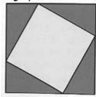
Figura 2: Una disección de un cuadrado de lado a + b
