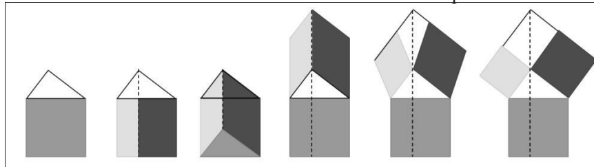
Figura 6: Demostración de Euclides – versión animada
