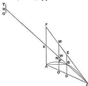
Figura 1: Sistema de la palanca de Arquímedes para “pesar” una región parabólica, extraído de Heath (1953).
