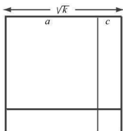
Figura 10: Disección de un cuadrado de área k
