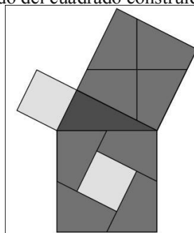
Figura 7: Disección de Perigal para demostrar el Teorema de Pitágoras
