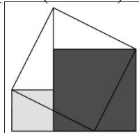
Figura 4: Una disección del cuadrado sobre la hipotenusa, de Thabit Ibn Qurra
