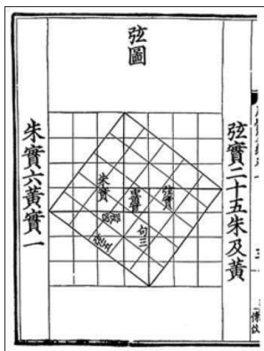
Figura 3: La “Figura de la hipotenusa”, acorde a la edición de 1213 de Zhoubi suanjing
